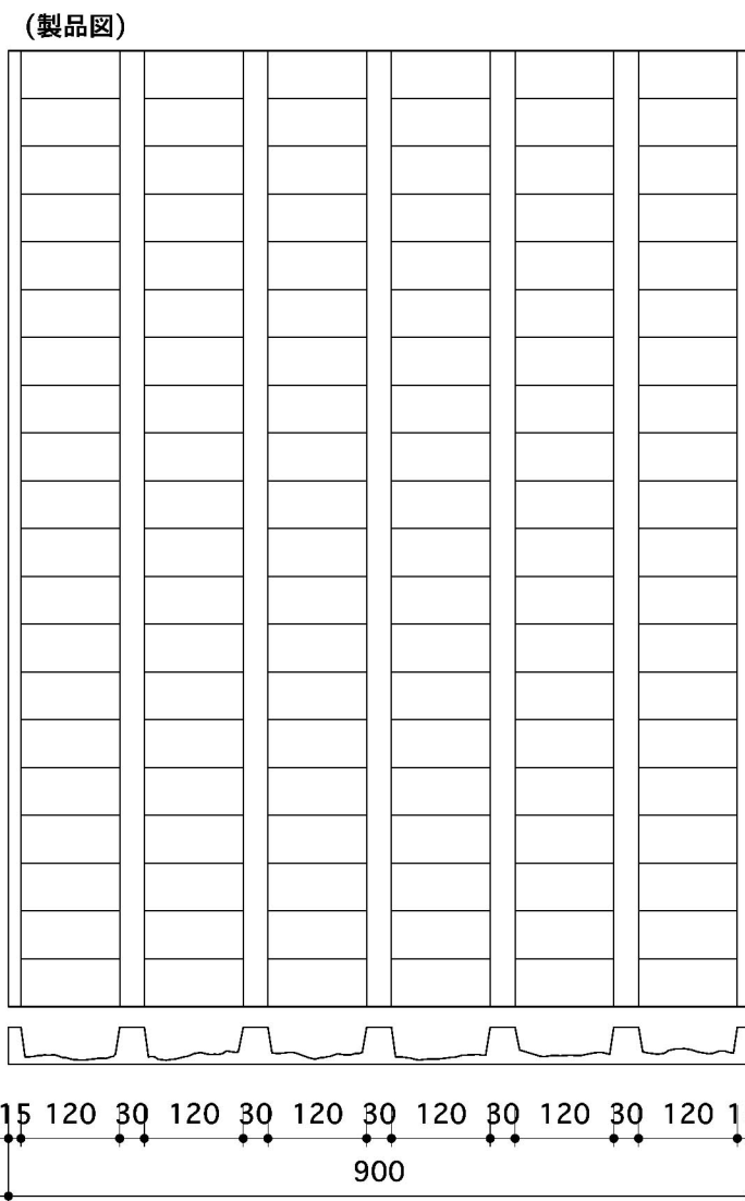
(仕上がり図)
